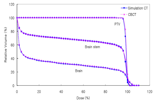
그림 13. Comparison of the DVHs for the brain tumor
