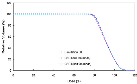
그림 12. Comparison of the target DVHs in the Catphan-600 phantom
