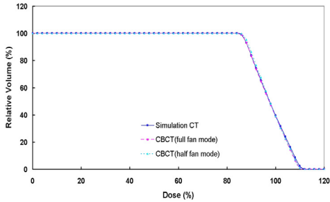
그림 11. Comparison of the target DVHs in the homogeneous phantom
