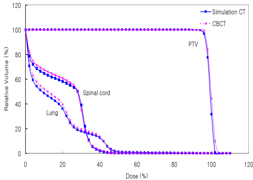
그림 14. Comparison of the DVHs for the lung cancer
