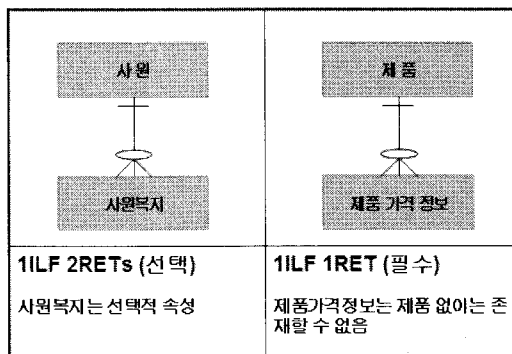
그림 2. RET 산정 예제 Fig 2. Calculation Example of RET
