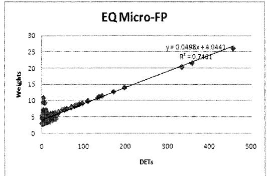
그림 4. 기능유형별 기능점수 회귀식 Fig. 4 Regression of FP by Function Type
