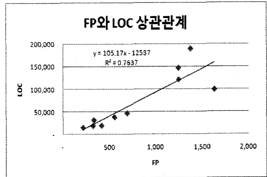
그림 5. IFPUG FPA와 LOC 상관관계 Fig. 5 Correlation of IFPUG FPA and LOC
