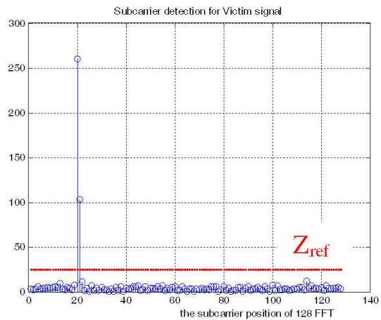
그림 9. Subcarrier 위치 추적 알고리즘의 시뮬레이션 예제 Fig. 9. A simulation example of the proposed algorithm to follow up the subcarrier position of victim signal.
