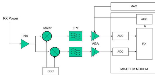
그림 3. VGA 조절 구조 Fig. 3. A structure for VGA control.
