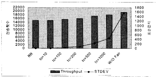
그림 7. 시뮬레이션 결과
