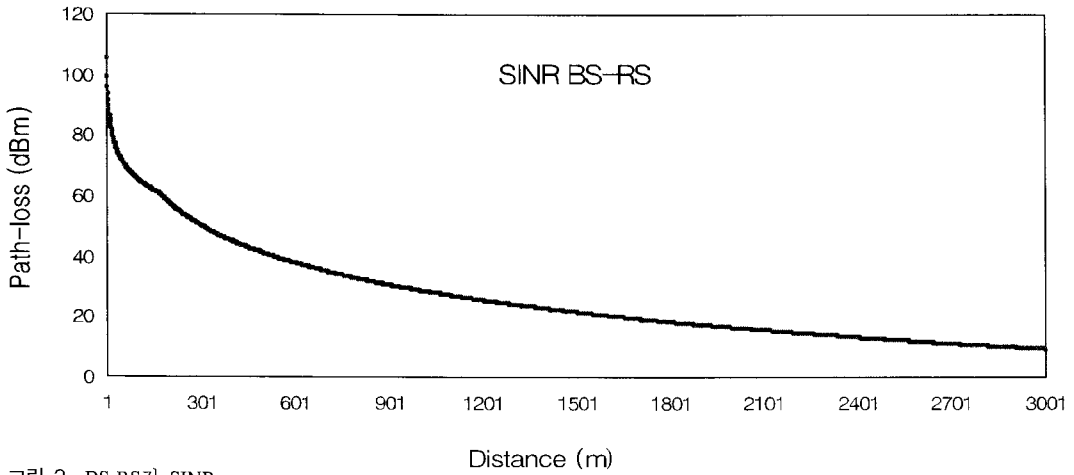
그림 3. BS-RS간 SINR
