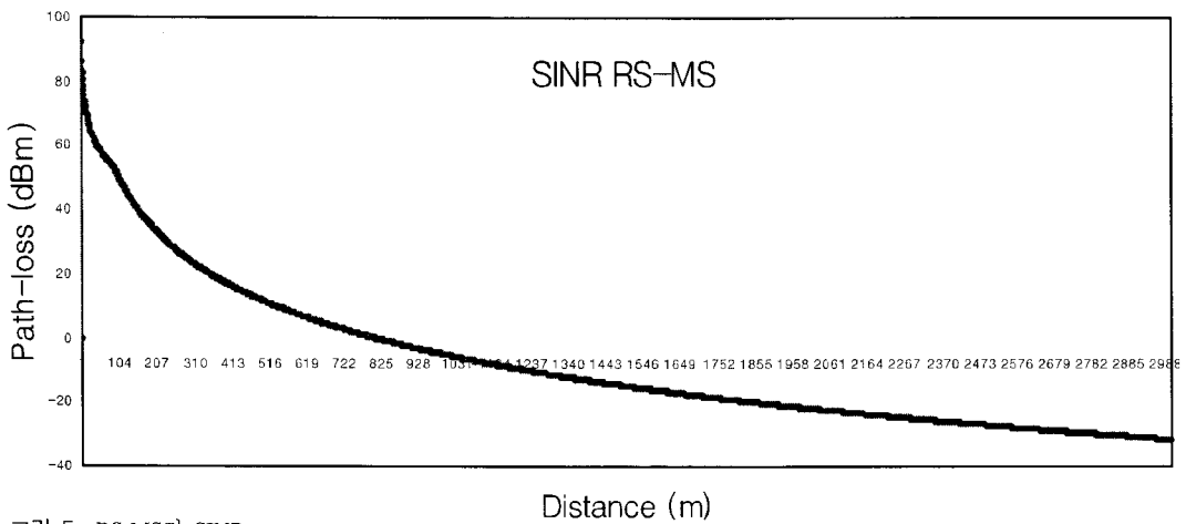
그림 5. RS-MS간 SINR
