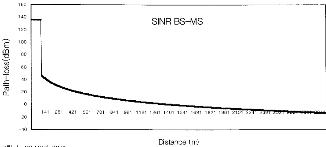
그림 4. BS-MS간 SINR
