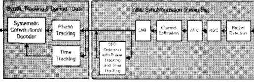
그림 3. 수신 동기 알고리즘 블록 다이어그램 Figure 3. Receive algorithm block diagram
