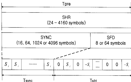
그림 2. SHR 프리앰블 구조 Figure 2. The Structure of the SHR Preamble
