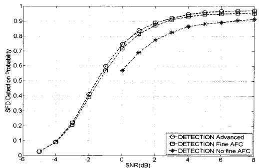
그림 9. 여러 방법에 따른 SFD 검출 확률 Figure 9. SFD Detection Probability vs. SNR for different method
