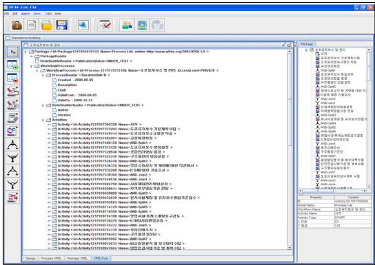
(그림 7) 예제 시나리오의 ICN 정형 노테이션 및 XPDL 정의
