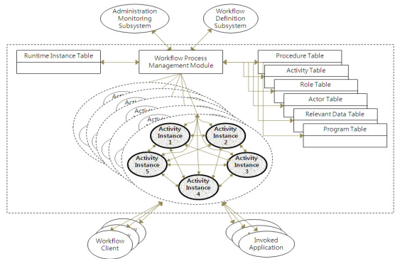
(그림 3) 동적 인스턴스 액티브 유형의 액티비티 인스턴스 기반 워크플로우 아키텍처
