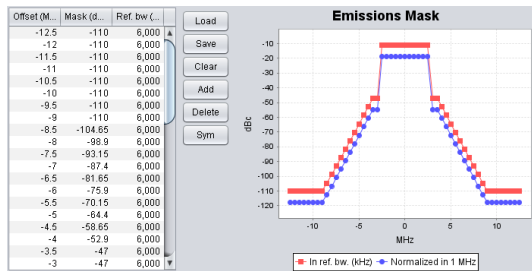
그림 4. CR 사용자 마스크 설정
