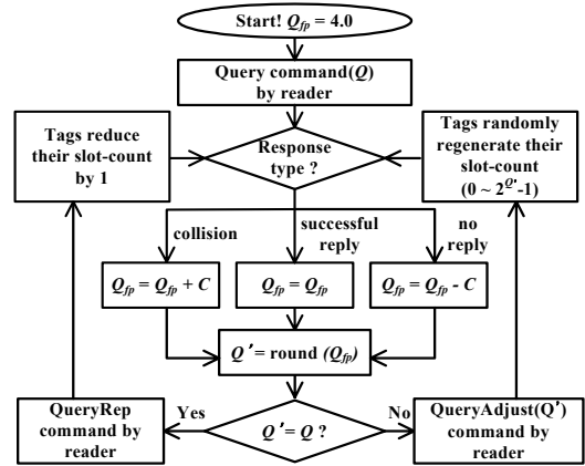
그림 1. 다중 태그 환경에서 리더가 태그를 인식하는 순서도
