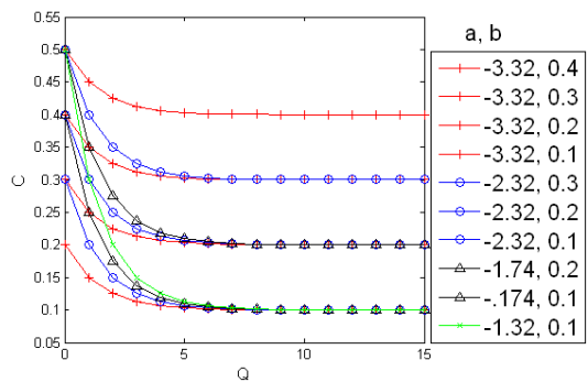
그림 4. 수식 C = A^{-Q} + a + b 에서 a 값과 b 값의 변화에 따른 지수 C 모델
