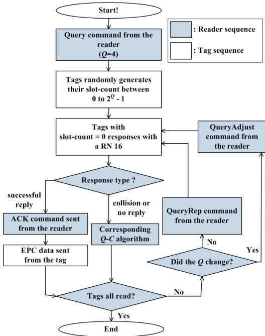
그림 5. 다중 태그 인식 성능 평가를 위한 시뮬레이션 모델의 흐름도
