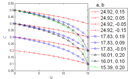
그림 3. 수식 C = \log_4(-Q + a) + b 에서 a 값과 b 값의 변화에 따른 log C 모델
