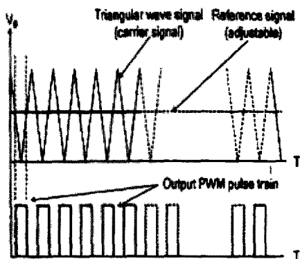
(b) MPWM
