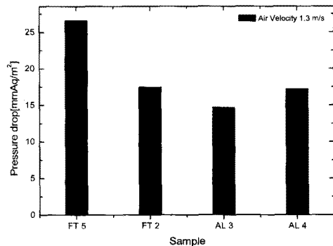
[그림 13] 대표 열교환기의 공기측 압력강하
