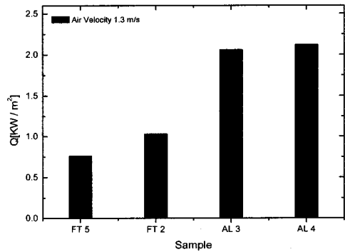
[그림 9] 대표 열교환기의 단위면적당 전열량
