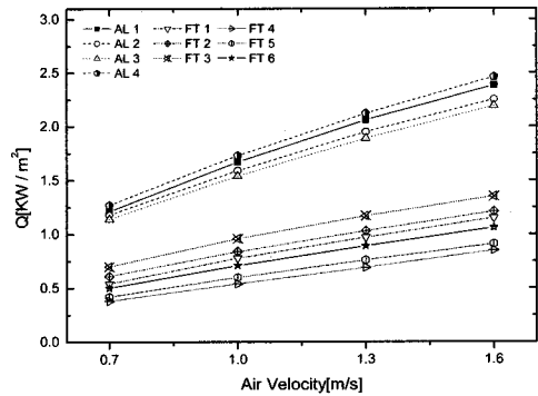
[그림 8] 전체 열교환기의 단위면적당 전열량
