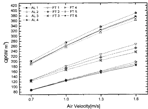
[그림 4] 전체 열교환기의 단위체적당 전열량
