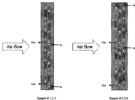
[그림 2] 실험에 사용된 핀-튜브 열교환기 개략도
