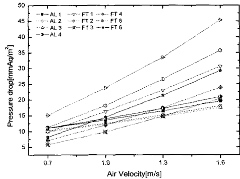
[그림 12] 전체 열교환기의 공기측 압력강하
