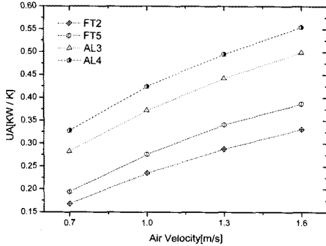
[그림 10] 대표 열교환기의 총괄열전달계수(UA)
