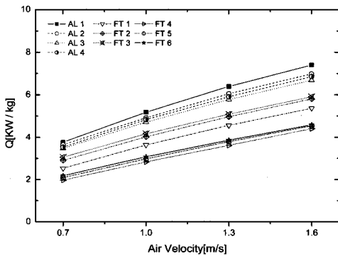
[그림 6] 전체 열교환기의 단위질량당 전열량
