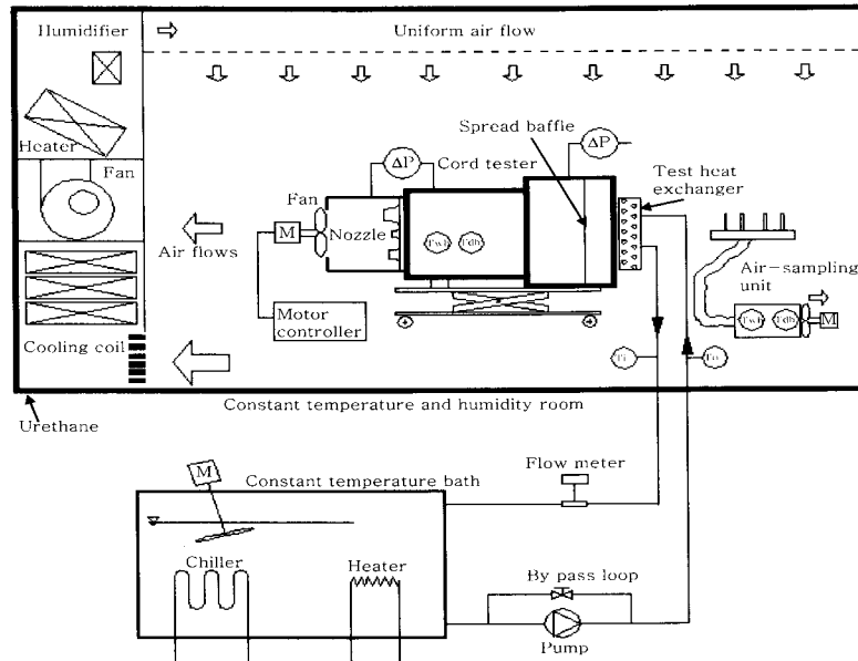
[그림 1] 실험장치 개략도
