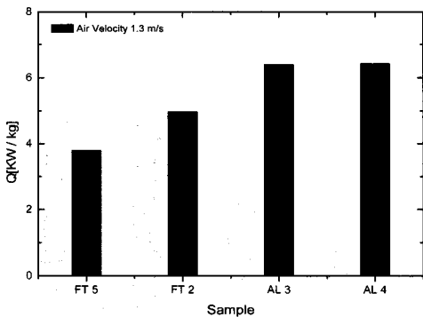
[그림 7] 대표 열교환기의 단위질량당 전열량
