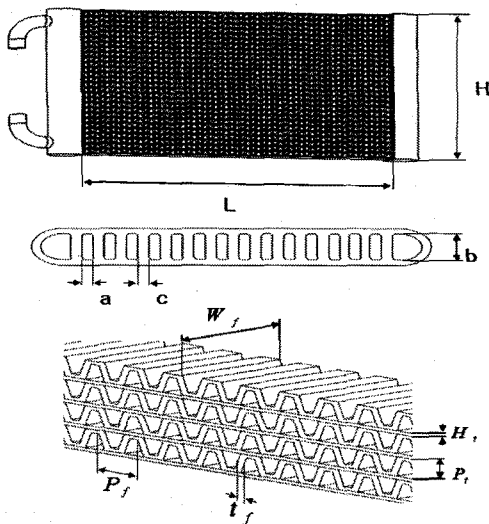
[그림 3] 실험에 사용된 알루미늄 열교환기 개략도
