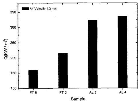
[그림 5] 대표 열교환기의 단위체적당 전열량
