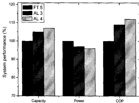
[그림 11] 대표 열교환기의 공조사이클 적용시 성능비교
