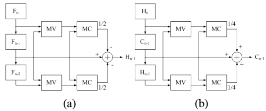
그림 6. MCTF의 구조 (a) 예측 (b) 갱신 Fig. 6. MCTF architecture (a) predict (b) update
