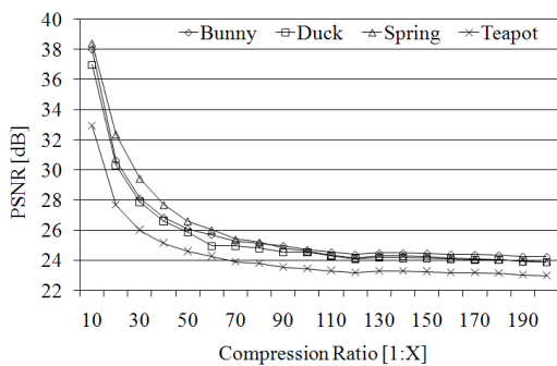
그림 8. 디지털 홀로그램의 PSNR 결과 Fig. 8. PSNR result of the compressed digital hologram
