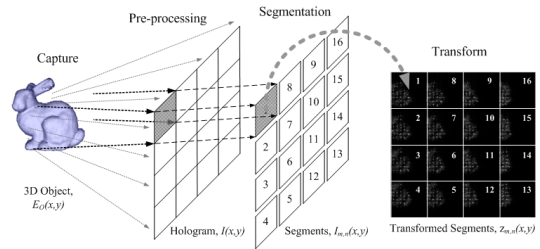
그림 3. Fringe pattern의 분할 및 변환 Fig.3. Segmentation and transform of fringe pattern
