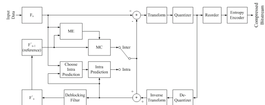
그림 7. H.264의 인코더 구조 Fig. 7. Encoding Architecture of H.264
