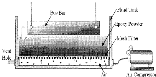
그림 2. 에폭시 분체도료의 실험장치.
