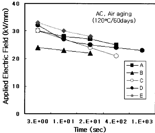
(a) 공기중 열화 (a) Degradation in air
