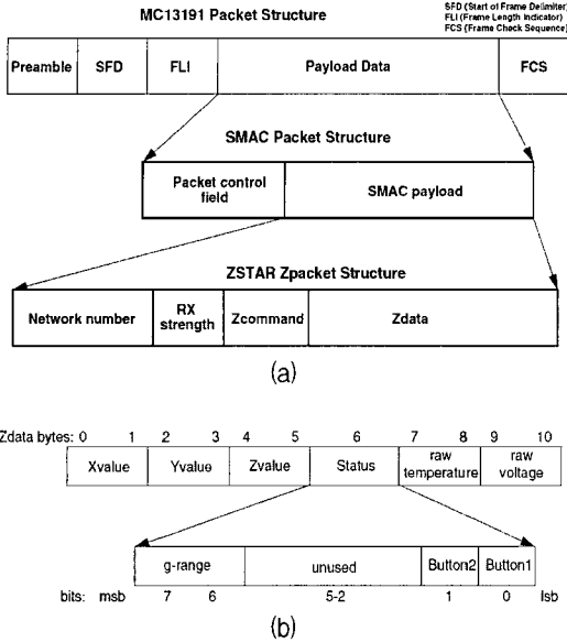
그림 4. ZSTAR Zpacket 구조 (a) Packet 구조 (b) Zdata 구조 Fig.4 Construction of ZSTAR Zpacket. (a) Packet Construction (b) Zdata Construction
