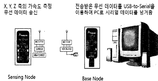
그림 1. 시스템 구성도 Fig. 1. System Configuration.
