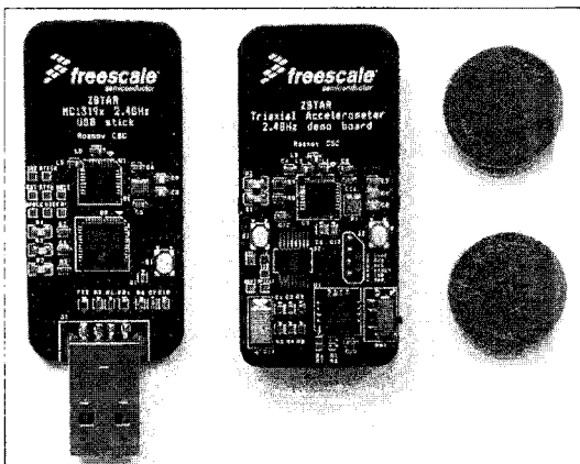
그림 3. 실험에 사용한 무선 센서 모듈 Fig.3 Wireless Sensor Module for Experiment.
