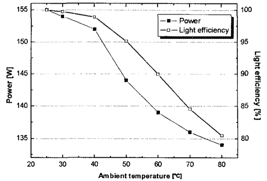
그림 8. 주변온도 증가에 따른 전력과 광효율.
