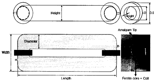
그림 1. 등근형 무전극 램프.
