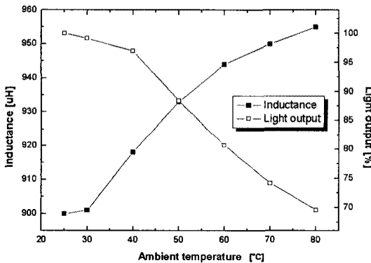
그림 7. 주변온도 증가에 따른 인덕턴스와 광출력 특성.
