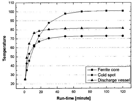
그림 4. 페라이트 코어와 방전관, 냉점의 온도변화. Fig. 4. Change of temperature in ferrite core and discharge tube and cold spot.
