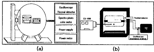
그림 2. 실험 개략도.
