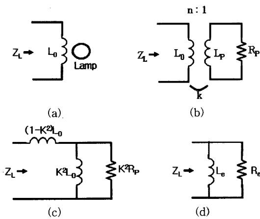
그림 3. 등근형 무전극 램프의 등가회로. Fig. 3. Equivalent circuit of cylinder type electrodeless lamp.
