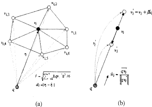
그림 4. (a) 임의의 v_i 와 q 에 인접한 꼭지점 v_{i,j} ( j \in [1, 6] )들과 기준점 q 와의 거리 차이 d_i = |r_i - \hat{r}_i| , (b) 꼭지점 v_i 를 \overrightarrow{qv_i} 방향으로 이동
