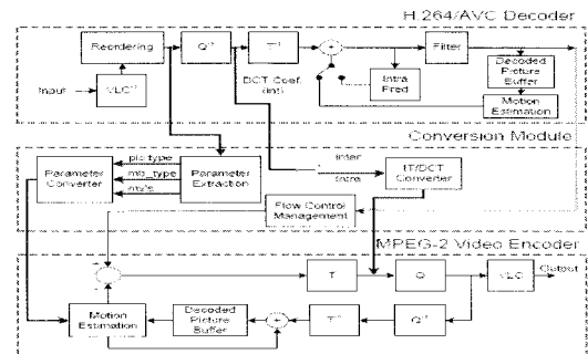
그림 2. 트랜스코딩 구조도
