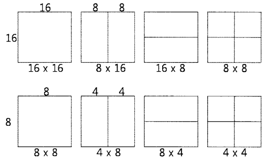
그림 1. H.264 매크로블록 파티션
