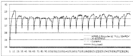
그림 7. Container영상의 PSNR비교
