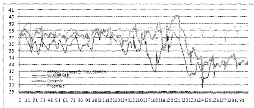
그림 9. FOREMAN영상의 PSNR 비교
