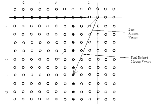
그림 3. 움직임벡터 정교화 방법
