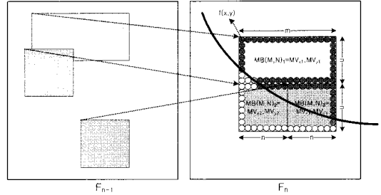
그림 5. 비용함수 및 예측움직임벡터 결정
