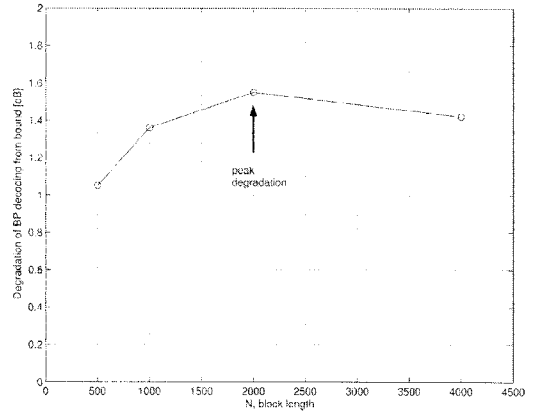
그림 3. 10^{-5} 의 BER에서 성능 한계로부터 BP 복호의 E_b/N_0 dB 성능 감쇠와 N=2000 에서 정점 성능 감쇠 (peak degradation)
