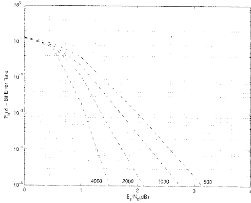
그림 1. BP 복호 성능 ( N = 4000, 2000, 1000, and 500. )
