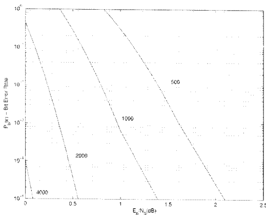
그림 2. 성능 한계 ( N = 4000, 2000, 1000, and 500. )
