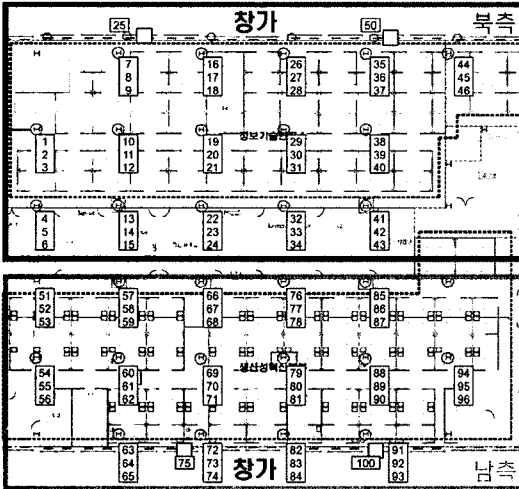
(그림 3) ASHRAE 표준에 준한 수평 배치 (창측으로부터 세가지 거리에 센서를 설치하였다.)
