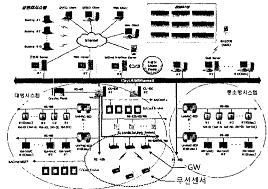
(그림 1) Control City의 시스템 구성도 및 무선 센서 도입 위치 (반투명 타원으로 표기한 부분이 과제 범위이다)
