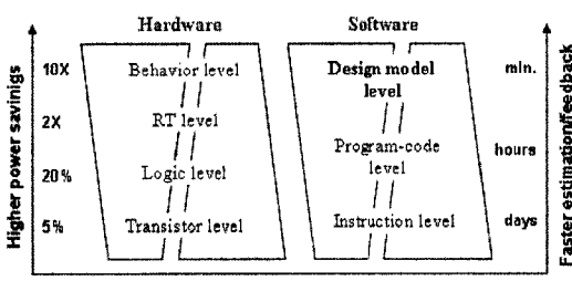
(그림 2) 추상화수준에 따른 소모전력분석 특성[2]
