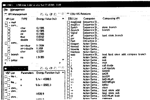
(그림 6) 에너지 라이브러리 화면
