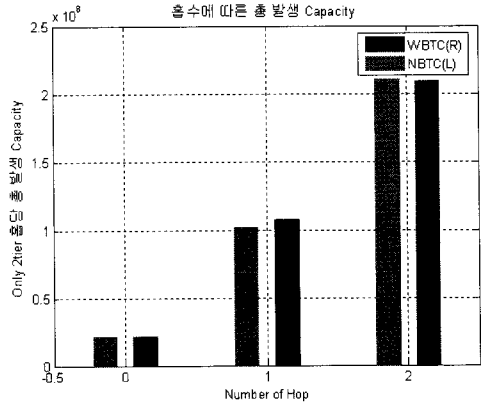
그림 12. NBTC 사용 셀 클러스터(좌측 막대)와 WBTC 사용 셀 클러스터(우측막대)의 총 용량 (Type D)
