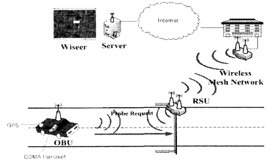
그림 3. 식별 및 위치 추적 서비스를 위한 시스템 구성도
