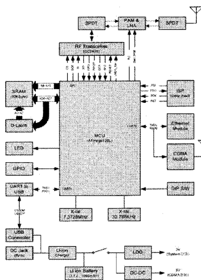
그림 4. 센서 게이트웨이 하드웨어 구조 Fig. 4. Sensor Gateway Hardware Architecture
