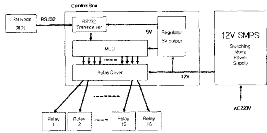
그림 6. 제어 노드 하드웨어 구성도 Fig. 6. Control Node Hardware Architecture
