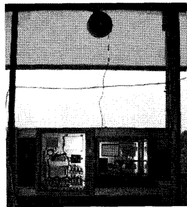
그림 7. 축사에 설치된 웹 카메라, 센서 게이트웨이와 제어 노드의 사진 Fig. 7. Photograph of Web Camera, Sensor Gateway and Control Node in the Stockyard
