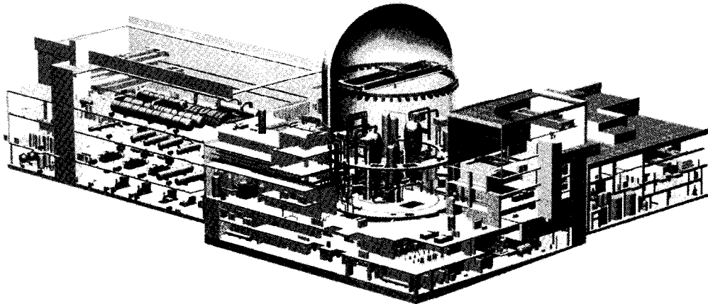
Fig. 1. APR1400 Cutaway
