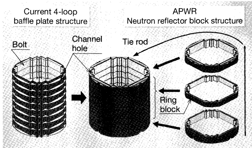
Fig. 3. Neutron Reflector
