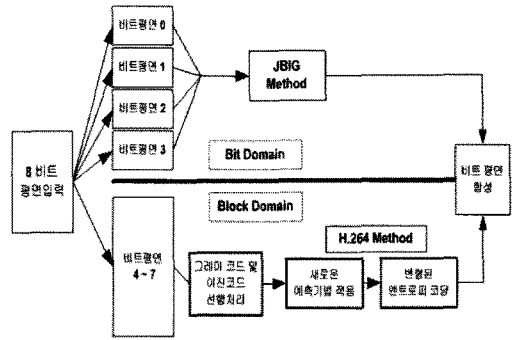
그림 2. 제안하는 부호화기의 구성
