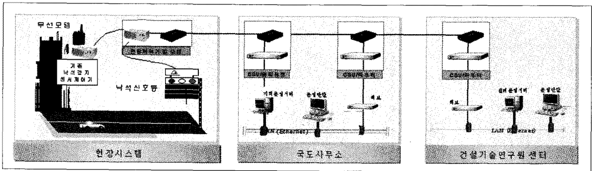
그림 8. 낙석신호등 구성도
