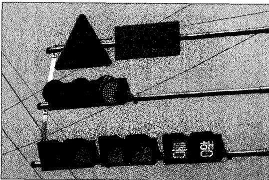
그림 9. 낙석신호등 설치 전경
