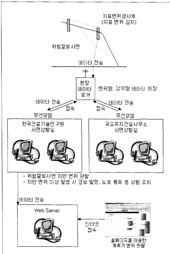
그림 5. 상시계측시스템 운용체계
