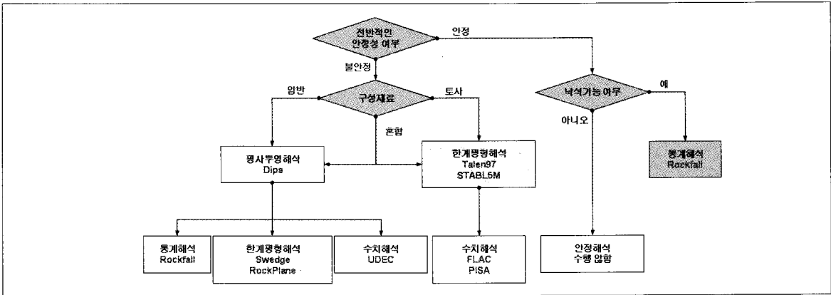
그림 4. 절토사면 구성 재료별 안정성 해석 수행 모식도
