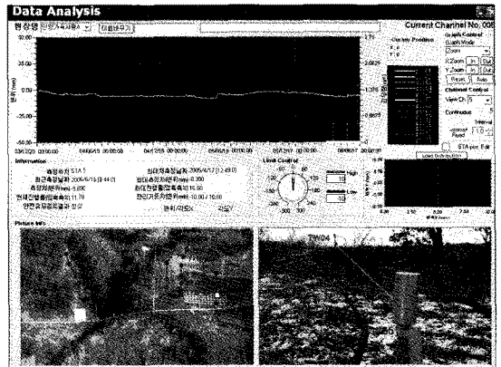
그림 6. 상시계측시스템 프로그램
