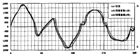
[그림 4] XP 8/16 롤러의 왼쪽지점 측정값
