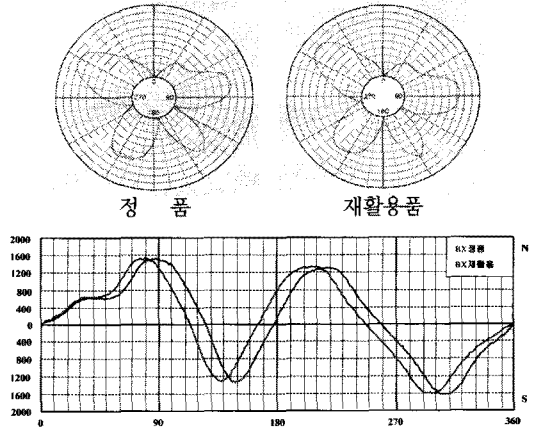
[그림 3] BX 롤러의 오른쪽지점 측정값
