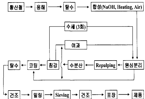
[그림 7] 제조공정
