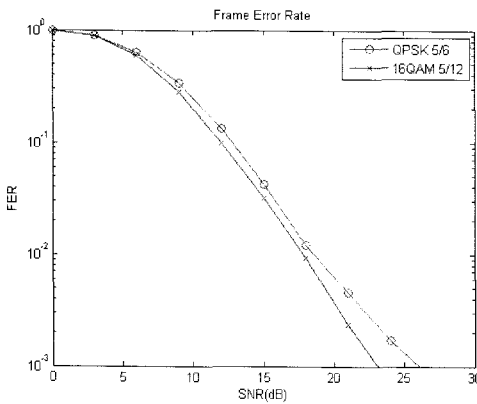
그림 2. 분산할당 SC-FDMA 시스템에서 위상회전 기술을 적용하였을 때의 성능
