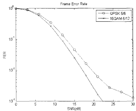
그림 4. 블록호핑 SC-FDMA 시스템에서 위상회전 기술을 적용하였을 때의 성능
