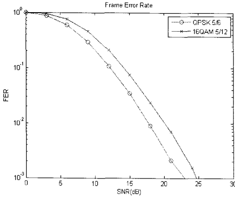
그림 1. 분산할당 SC-FDMA 시스템에서 순환지연 다이버시티를 적용하였을 때의 성능
