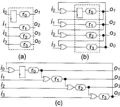
그림 7. 정규표현식 r^+ 에 대한 패턴 매칭 회로 (a) 패턴 r 에 대한 회로 (b), (c) 패턴 r^+ 에 대한 회로
