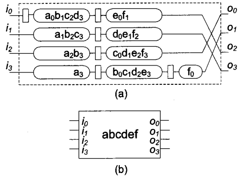
그림 5. 4바이트 단위 고정패턴 매칭 회로 (a) 내부 회로 (b) 블록도
