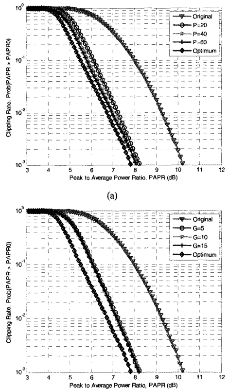
그림 6. 톤 수 K=1 이고, (a)세대 수 G=5 로 고정하고 개체 수 P 를 변화시킨 경우, (b) 개체 수 P=20 으로 고정하고 세대 수 G 를 변화시킨 경우에 대한 성능 비교
