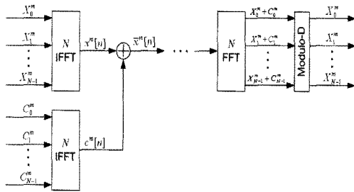
그림 2. 톤 삽입 기법을 위한 송·수신단 구조
