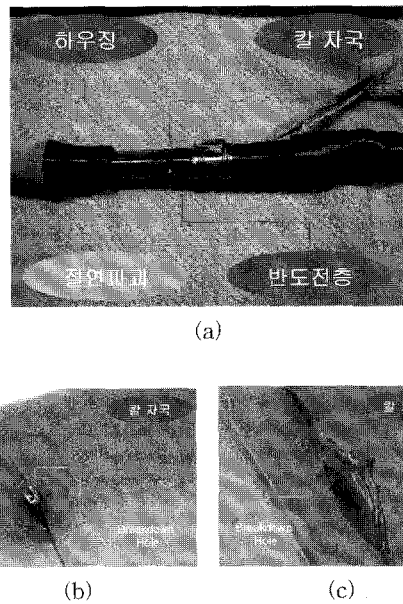
그림 7. 두께 감소에 따른 절연과피 위치 및 형상. (a) 위치, (b) 1 mm 감소, (c) 2 mm 감소.
