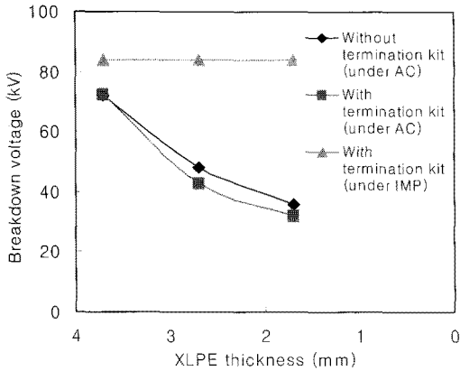
그림 6. 두께 감소에 따른 절연과피 전압. Fig. 6. Breakdown voltage depend on thickness decrease.
