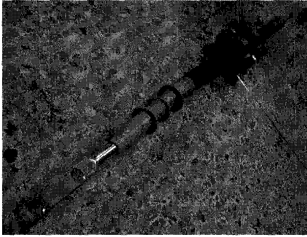
그림 3. 케이블 종단부 내전압 시험 시료. Fig. 3. Specimen for withstand test of cable terminal.
