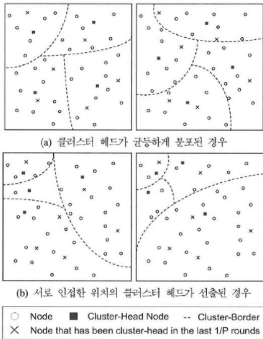
(그림 1) LEACH의 클러스터 구성 시나리오
