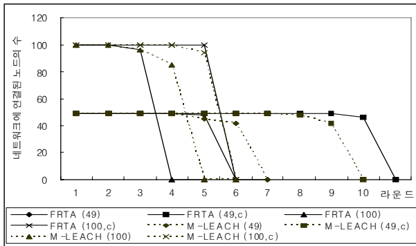
(그림 10) 네트워크 수명 비교
