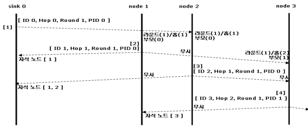
(그림 7) 라운드 패킷의 정방향과 역방향
