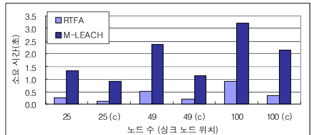
(그림 8) 라우팅 트리 구축시간 비교
