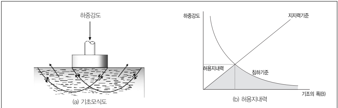
그림 5. 지지력과 침하 관계
