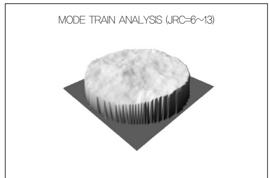
그림 4. 절리면 거칠기(JRC 레이저분석)
