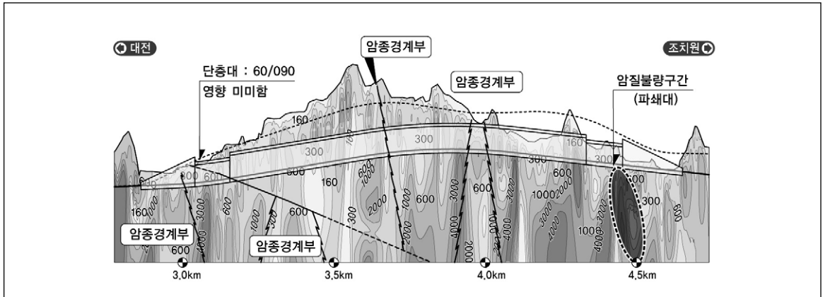
그림 2. 전기비저항 탐사결과
