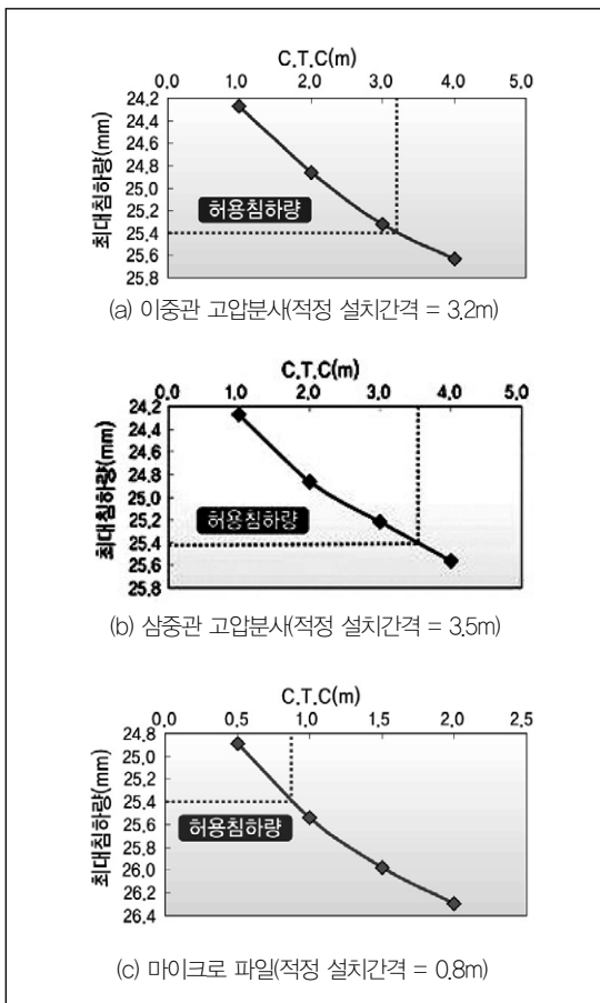
그림 9. 보강공법별 적정 설치간격
