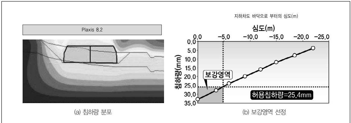
그림 8. 침하량 분포에 따른 보강영역 선정
