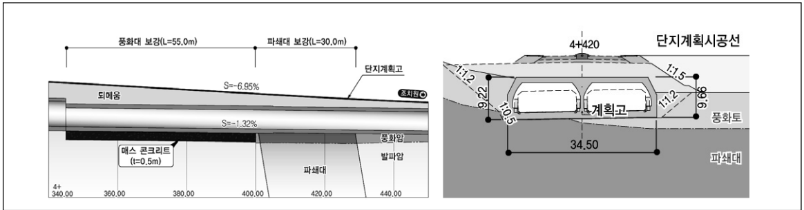
그림 6. 해석구간 및 대표단면
