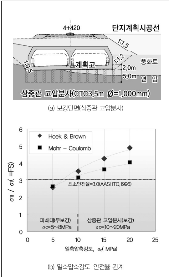
그림 10. 파괴규준을 이용한 보강효과 분석
