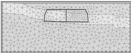
그림 7. 해석요소망(STA.4+420)
