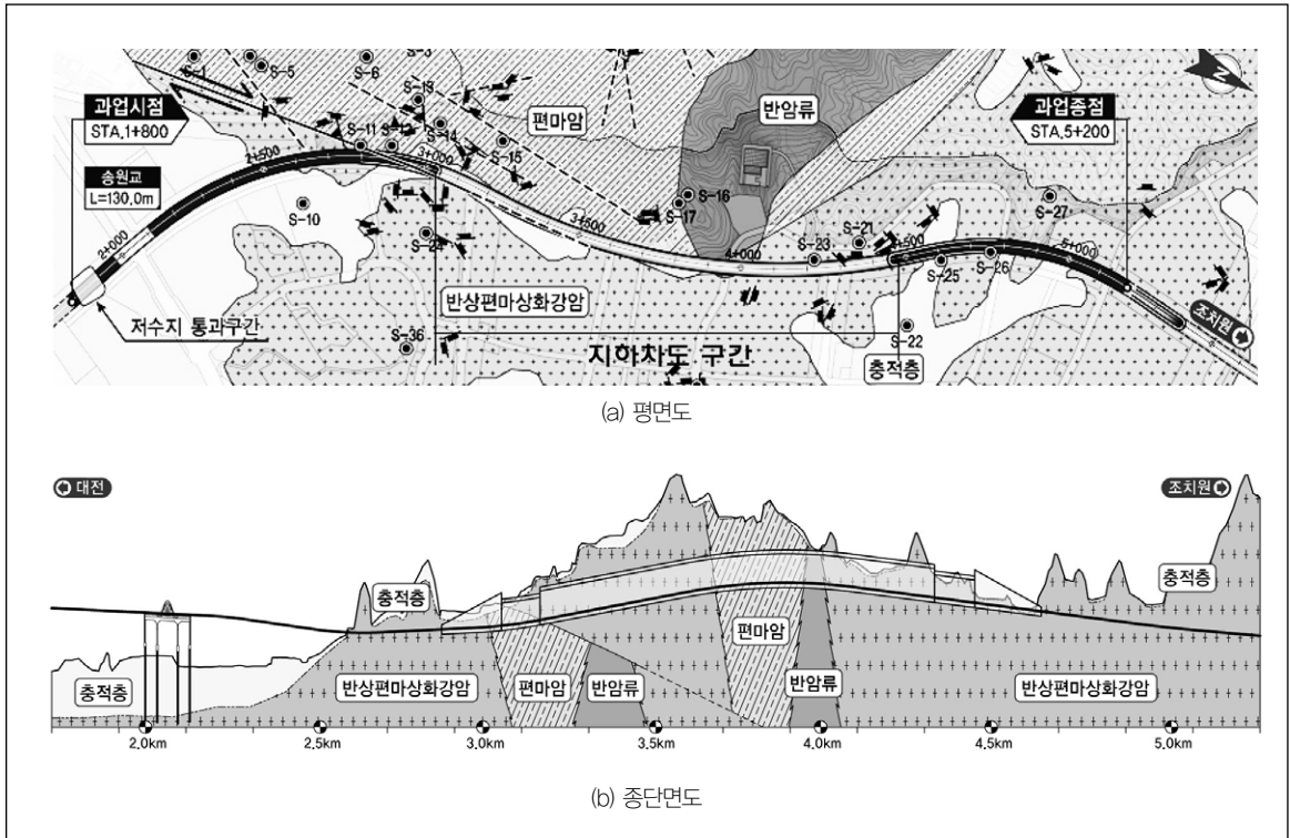
그림 1. OO지역 지질분포
