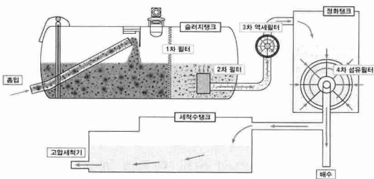
오수처리계통도
