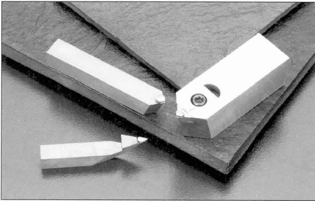
▶ 신진다이아몬드의 주력제품인 초정밀 코아 금형가공용 다이아몬드 바이트
