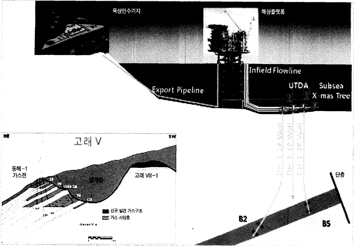
그림 11 동해-1 가스전 개발 모식도
