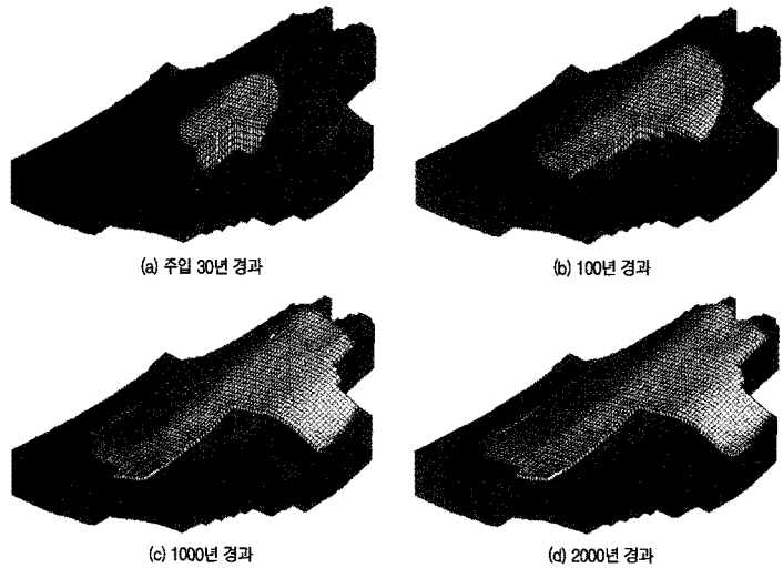
그림 9 동해-1 가스전 CO2 저장 시뮬레이션 사례
