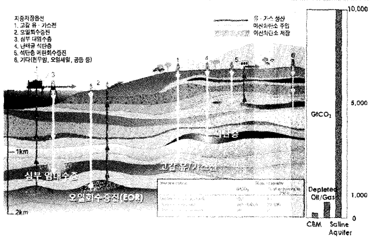
온실가스 지중저장방법 및 추정용량(IPCC)
