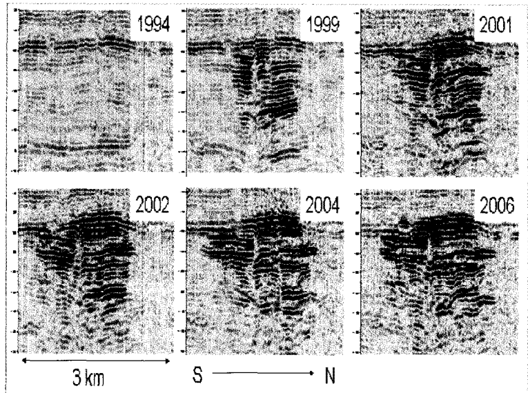
그림 8 탄성파탐사에 의한 이산화탄소 거동 모니터링(슬라이프너)
