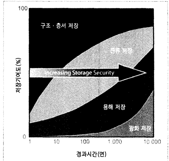
그림 4 지중저장 메커니즘 및 안정성(IPCC)
