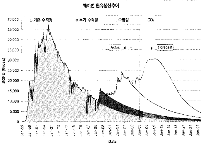
그림 7 CO 2 주입에 의한 회수율 증진(웨이번 사례). (BOPD: 하루 오일 생산량, 배럴)
