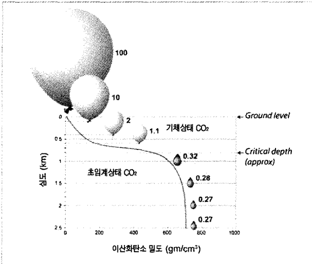
그림 3 심도에 따른 이산화탄소의 밀도 변화
