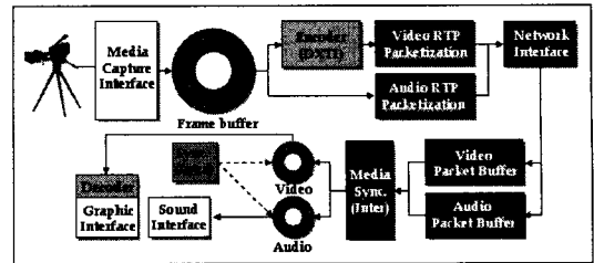
그림 4. 시스템 구성도
