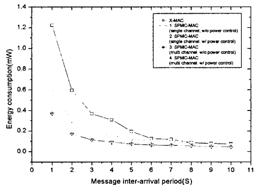
그림 7. SPMC-MAC과 X-MAC의 에너지 소모 비교 (Message inter-arrival time, packet size of 50 bytes.)
