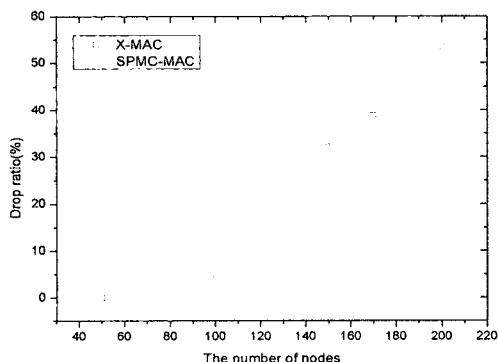
그림 10. SPMC-MAC과 X-MAC의 패킷 손실율(Packet drop ratio) 비교
