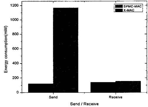
그림 4. 에너지 소모량 비교(SPMC-MAC/X-MAC)
