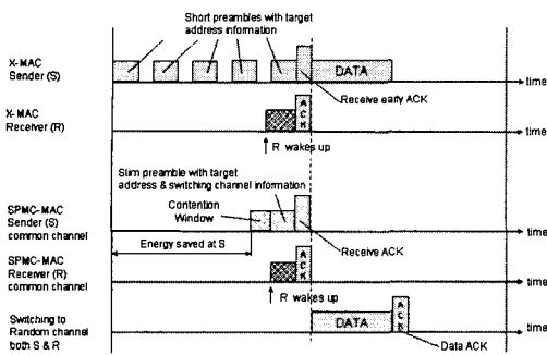
그림 1. SPMC-MAC(제안하는 맥)과 X-MAC 비교
