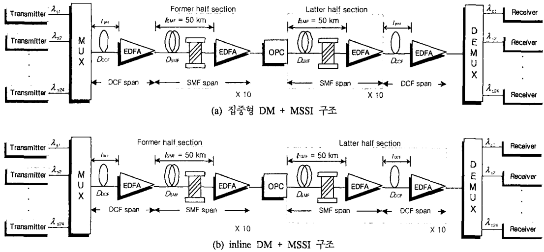
그림 1. 24×40 Gbps WDM 전송 시스템
