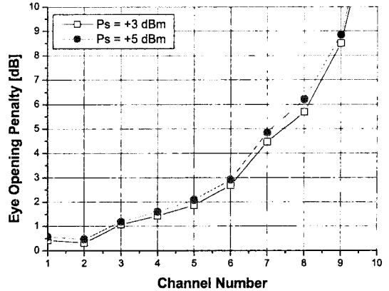
그림 3. WDM 전송 링크에 OPC만 적용한 경우의 채널에 따른 눈 열림 패널티
