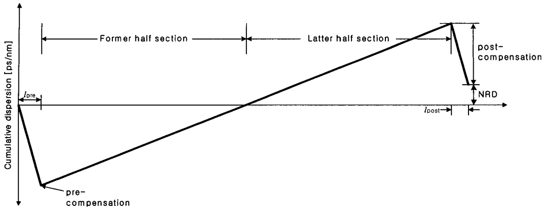
(a) 집중형 DM + MSSI 구조
