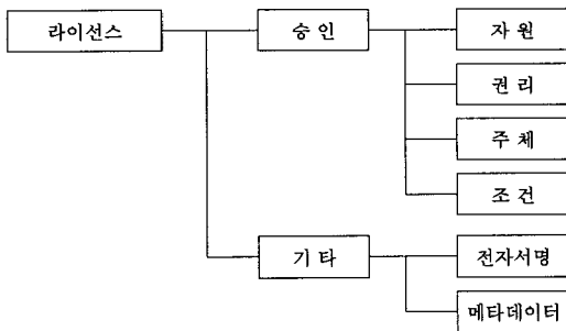
그림 1. 라이선스 구조도
