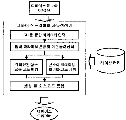
그림 3. 디바이스 드라이버 자동생성기 흐름도
