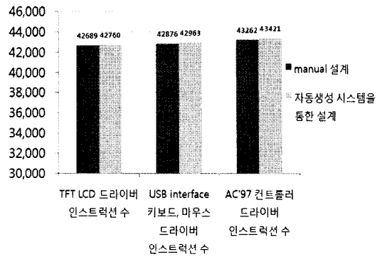
그림 7. 컴파일된 디바이스 드라이버의 인스트럭션 수
