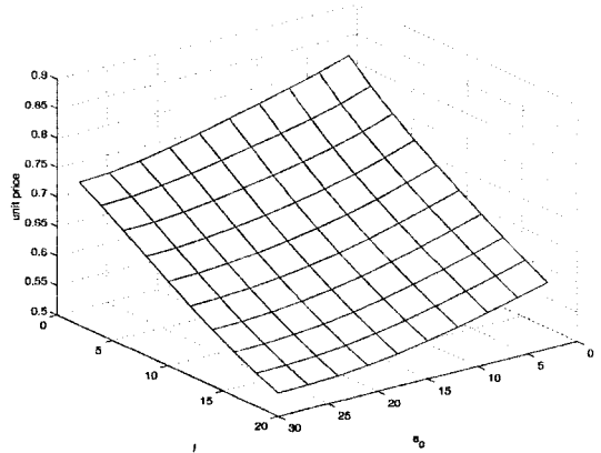
그림 2. a_0 와 l 의 함수로써의 단위 가격 ( C=50, \lambda=2, 1/\mu=50, T=110 )
