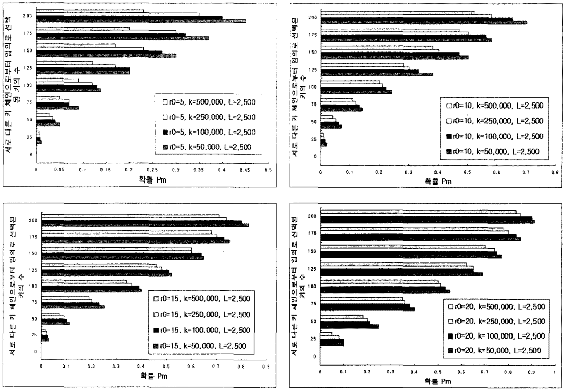
그림 2. 네트워크 크기가 n=10,000 일 때, 서로 다른 키 체인으로부터 임의로 선택된 키의 수( r_0, r_1 )와 확률 p_m 사이의 관계
