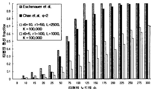
그림 4. n=10,000 , p_m=0.5 그리고 R = 168을 가지는 보안 강도
