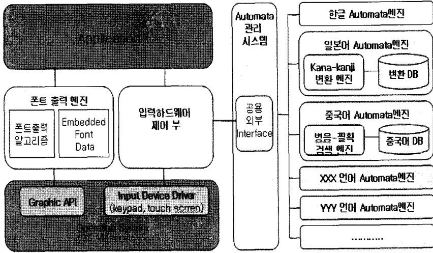
(그림 4) 한, 중, 일, 영 입력 시스템 구조도
