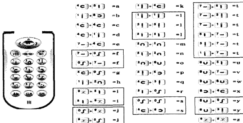
(그림 5) 영어 입력 오토마타
