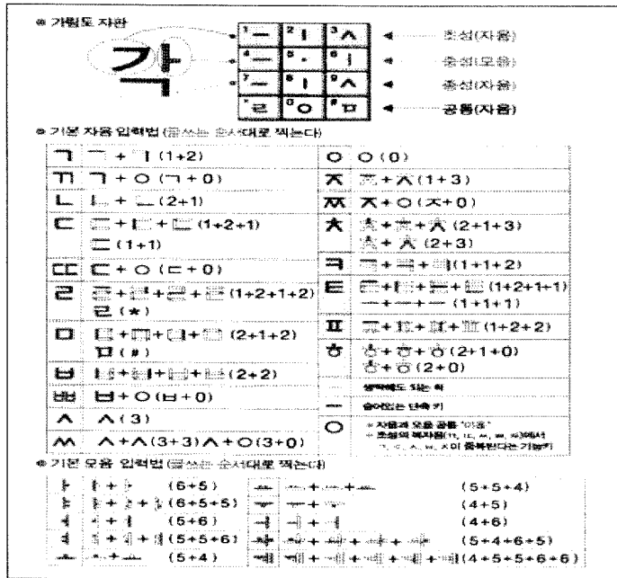
(그림 6) 한글 입력 오토마타
