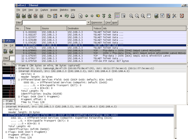
(그림 9) NGN 자원제어 테스트-베드에서의 IP 패킷의 DSCP 코드
