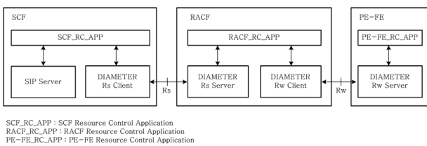
(그림 4) Rs와 Rw 인터페이스에서 DIAMETER의 클라이언트와 서버 관계
