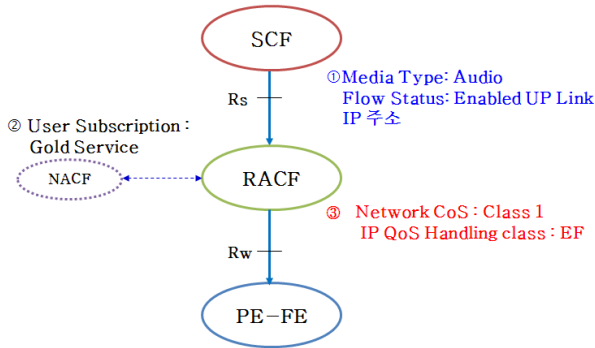
(그림 3) 네트워크 서비스 클래스와 IP QoS 핸들링 클래스 결정 단계
