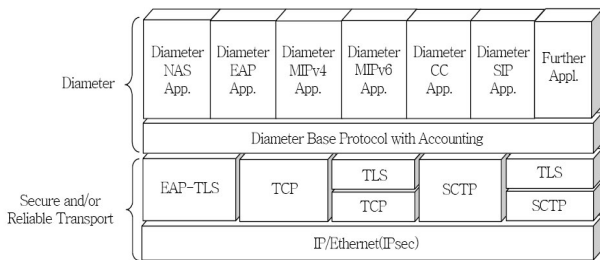
(그림 2) DIAMETER 프로토콜의 구조
