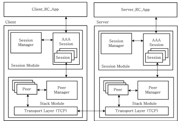
(그림 5) DIAMETER 기반 NGN 자원제어 프로토콜의 기능구조
