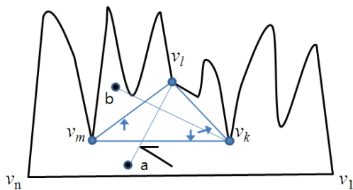
(그림 6) 세 번째 경우의 단변단조 다각형에 대한 증명
