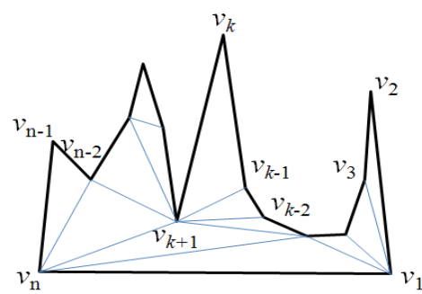
(그림 4) 단변단조 다각형과 삼각화의 예
