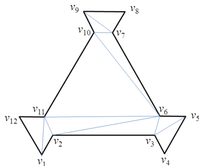
(그림 9) 완전외부가시성 다각형에서 GSS가 되는 삼각화의 예
