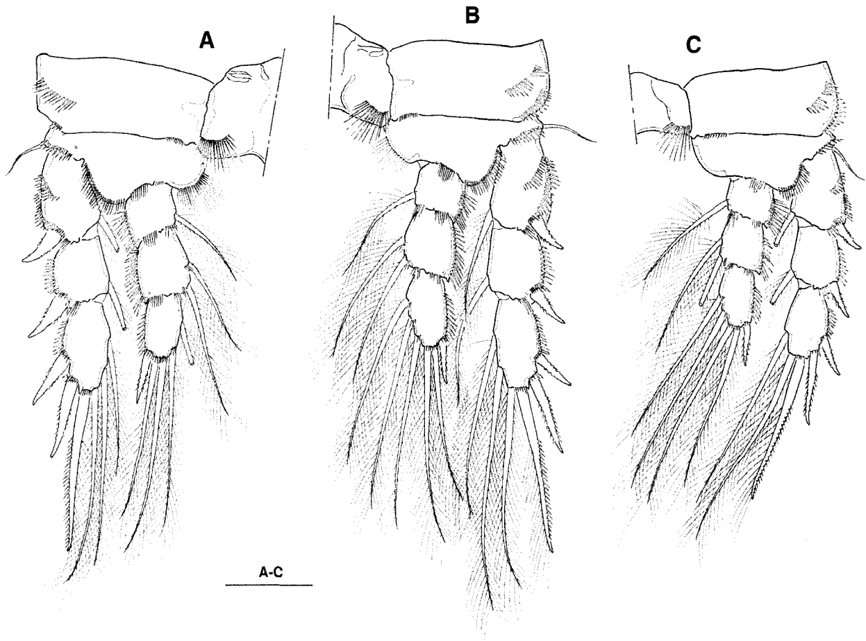
Fig. 7. Geeopsis incisipes (Klie), female. A, P2; B, P3; C, P4. Scale bar=50 µm.
