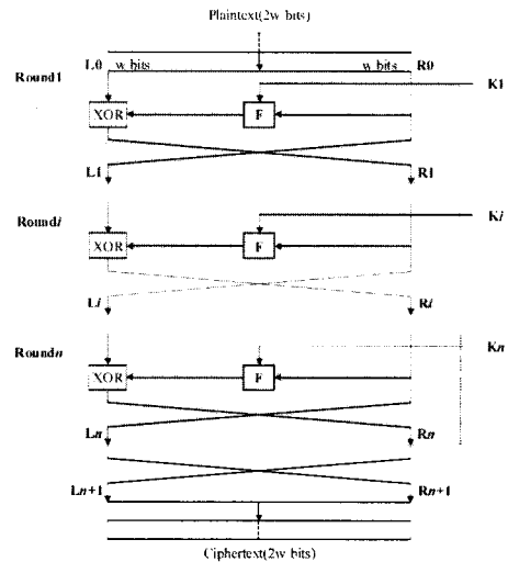
Fig 1. Feistel encryption structure 그림 1. Feistel 암호화 구조
