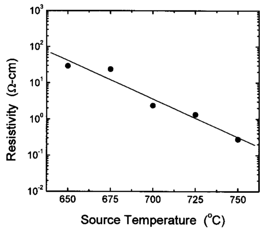
그림 6. 소스 온도에 따른 CdS 박막의 비저항.
