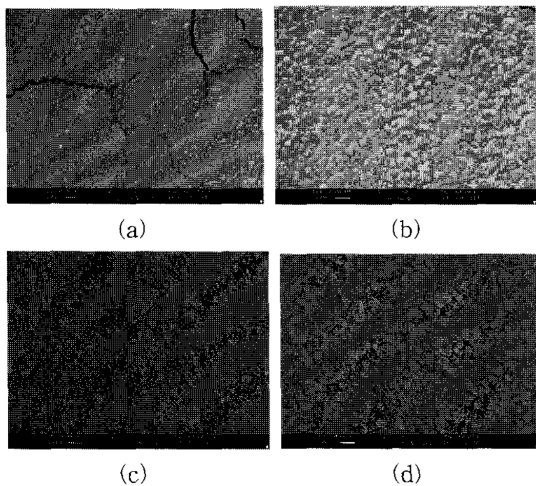
그림 8. 기판온도에 따른 CdS 박막의 미세구조: (a) T_s : 100 °C, (b) T_s : 150 °C, (c) T_s : 200 °C, (d) T_s : 250 °C.
