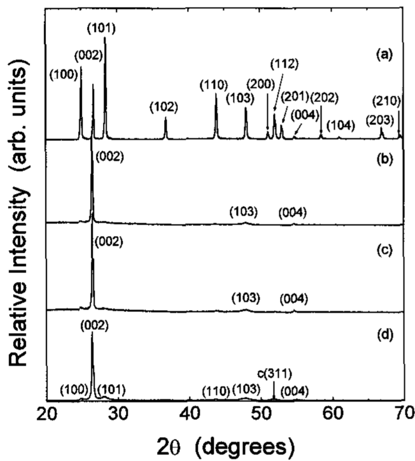
그림 2. 소스 온도에 따른 CdS 박막의 X-ray 회절 pattern: (a) CdS powder, (b) 650 °C, (c) 675 °C, (d) 750 °C.
