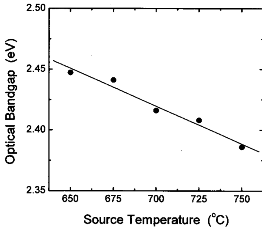
그림 5. 소스 온도에 따른 CdS 박막의 광학적 밴드 갭.
