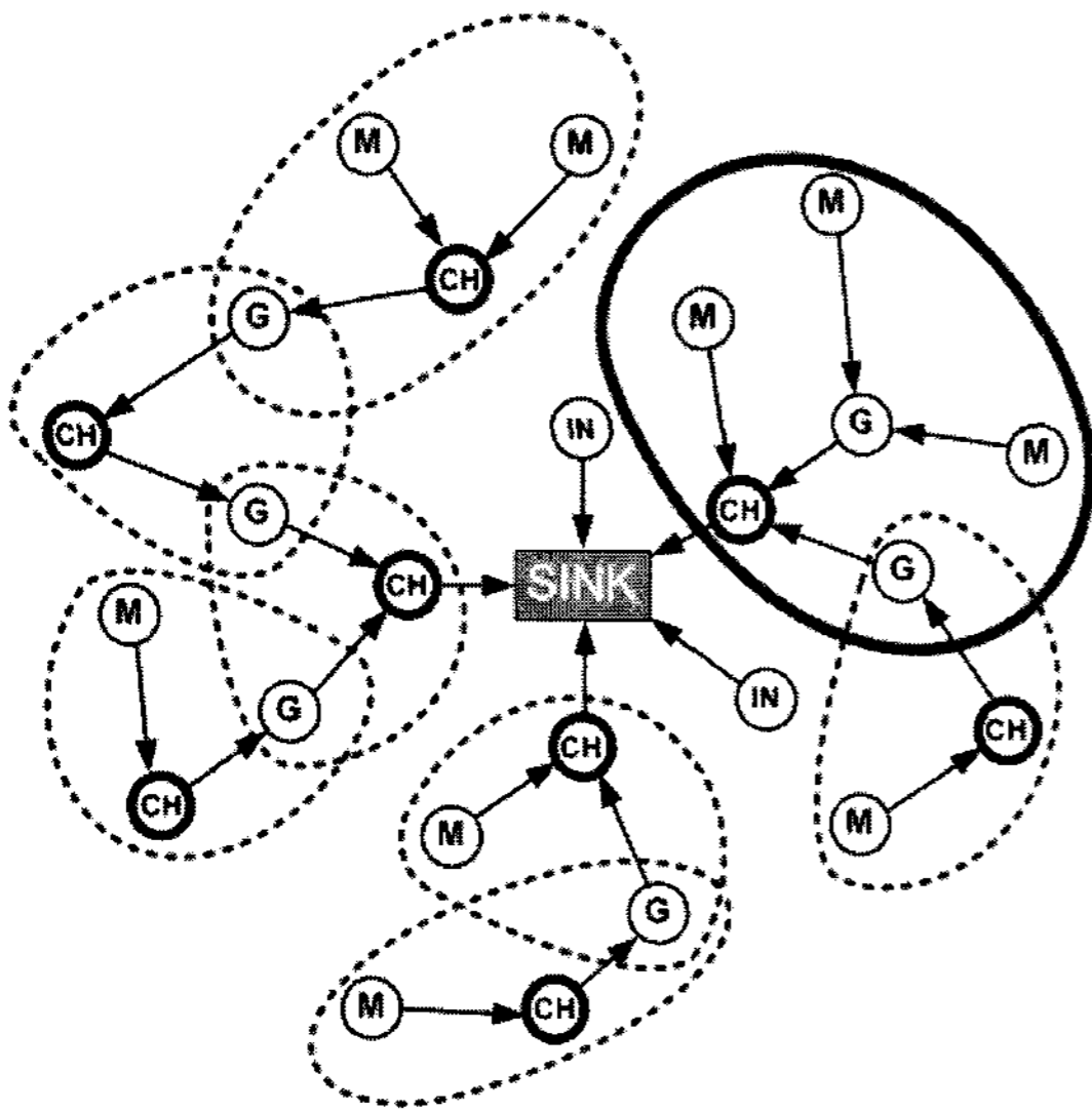
그림 6. 클러스터 구성 알고리즘 이후 경로 설정 Fig 6. Path Establishment after cluster configuration algorithm
