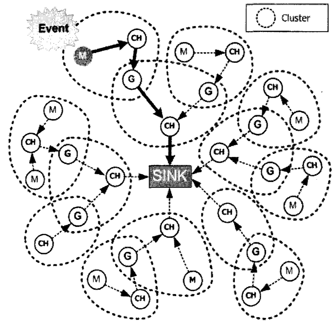
그림 2. 다수의 클러스터들로 구성된 무선 센서 네트워크 Fig. 2 The wireless sensor networks consisted of multiple clusters
