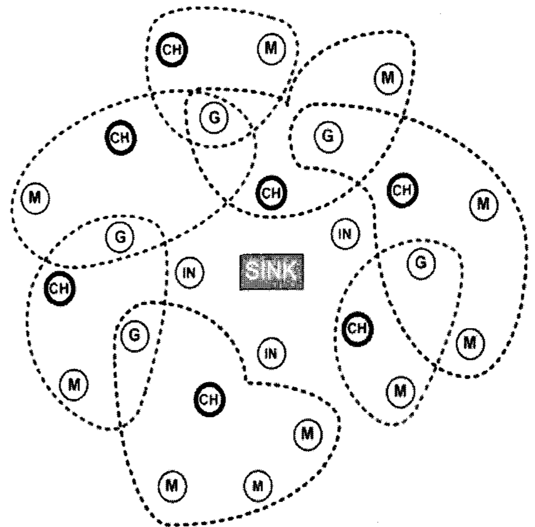
그림 5. 클러스터 재구성 이후에 네트워크 아키텍처 Fig 5. Network architecture after cluster reconfiguration
